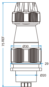
产品外型尺寸图 dimensions figure
