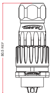
产品外型尺寸图 dimensions figure
